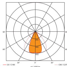
Fotometrijska krivulja LHBH
