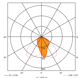
Fotometrijska krivulja RHISS
