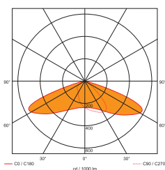
Fotometrijska krivulja LSJB
