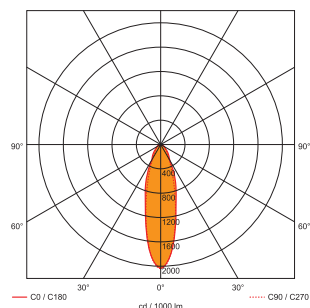
Fotometrijska krivulja RHIS30
