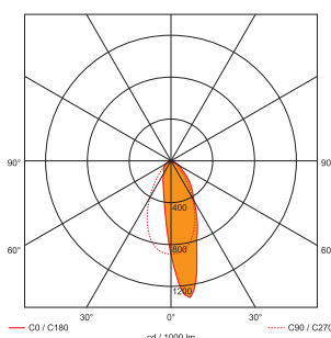
Fotometrijska krivulja RHISA
